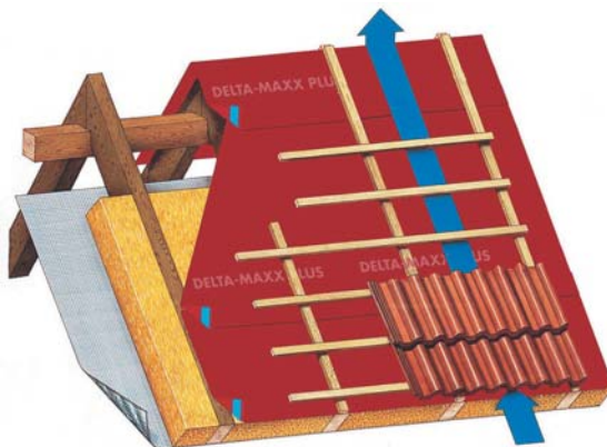
Schemat dachu z użyciem folii Delta®-Maxx Plus i Delta®-Reflex
