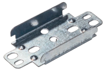
Wieszak bezpośredni do CD 60
