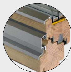
aluminiowy Classic (Softline / XL)
