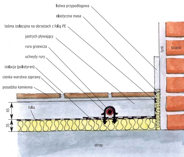
Przekrój przez podłogę z wodnym ogrzewaniem podłogowym
