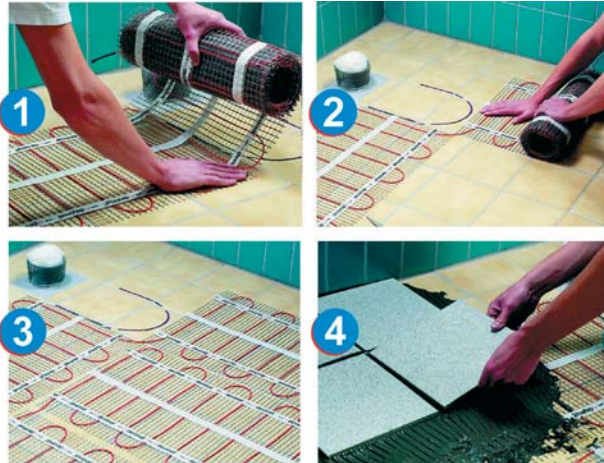
Etapy montażu maty grzejnej
