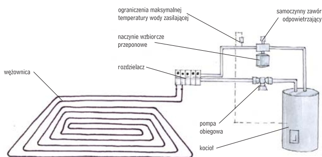
Ogrzewanie wodne z ogrzewaniem podłogowym zasilanym przez rozdzielacz
