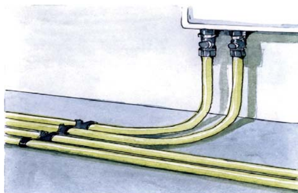
Mocowanie rur na szlifiec podłogowej
