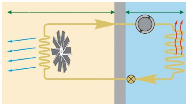
Budowa klimatyzatora
