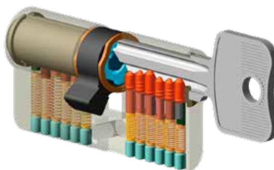
Wkładka klasy A
