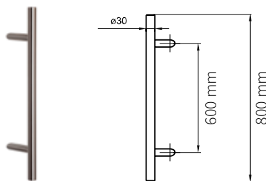
Zewnętrzny pochwyt prosty odgięty 45° (stal nierdzewna), długość 800 mm
