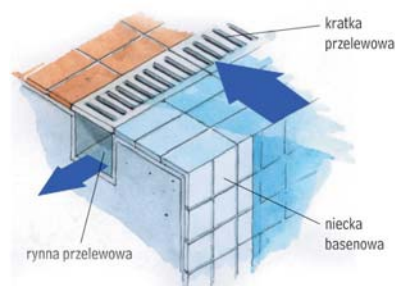
Zasada działania rynny przelewowej
