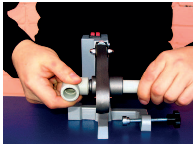
Rozgrzewanie rury Stabi FAST
