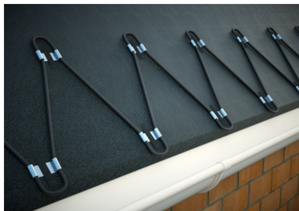
Uchwytów z blachy miedzianej lub cynkowo tytanowej
