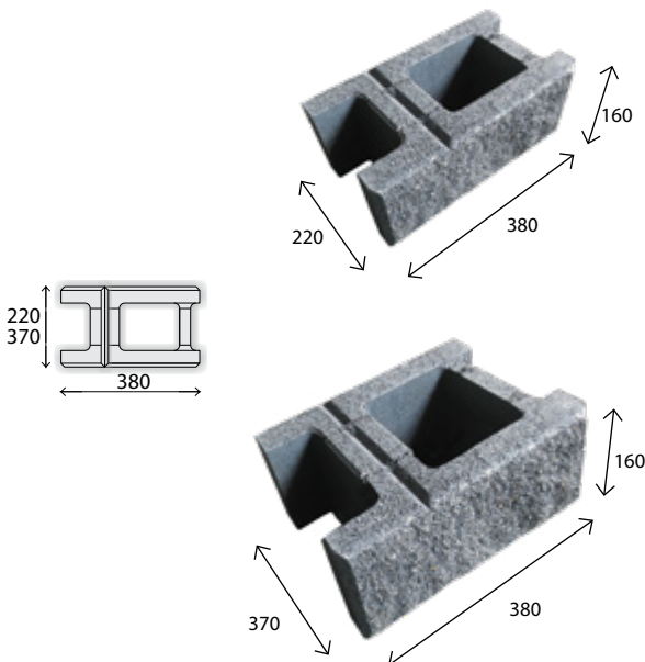
Bloczek cokołowy 370
