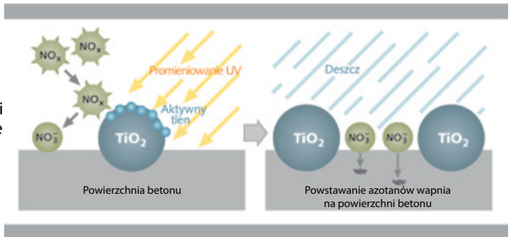
Mechanizm oczyszczania powietrza z tlenków azotu NO_x przez aktywną fotokatalityczną powierzchnię kostki brukowej wykonaną z użyciem cementu TioCem ®
