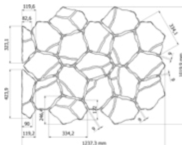
Ułożenie kostek Sasso
